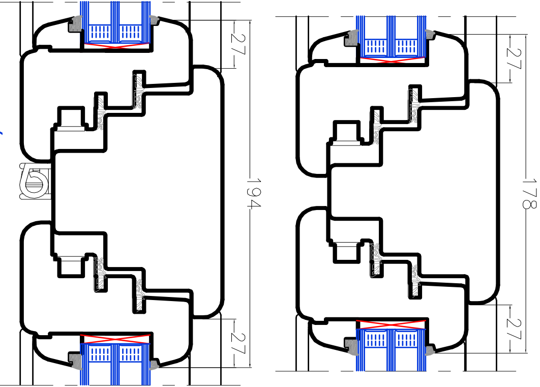
SZCZEGÓŁ A-A
